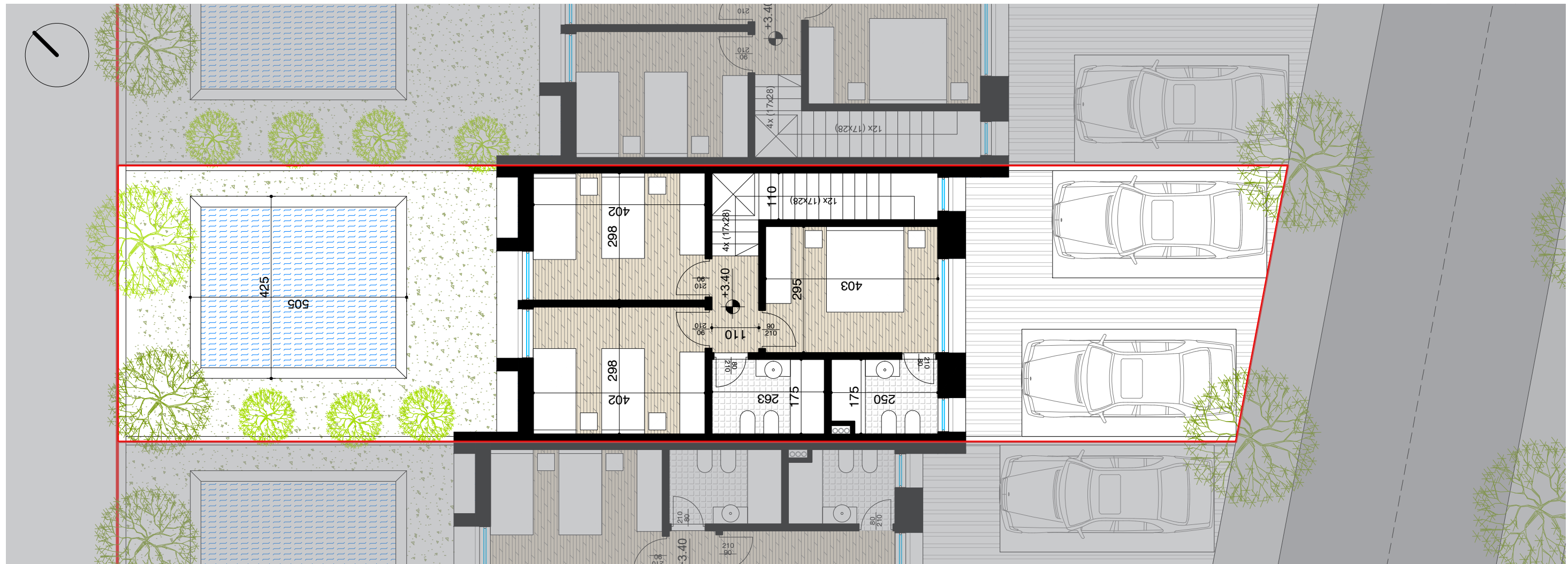
PLANIMETRI E KATIT TE PARE SH. 1:100
